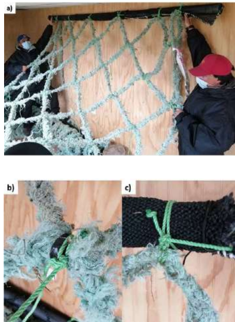
Figura 2: Armado del sistema BIVALNET® horizontal (BH). a) BH formato de 50cm, b) Puntos de unión de la malla con cabo PP Ø 5mm, c) Punto de unión del tramado a tubos HDPE con cabo PP Ø 5mm y malla de red de pesca anchovetera. Nota: Ø=diámetro.
