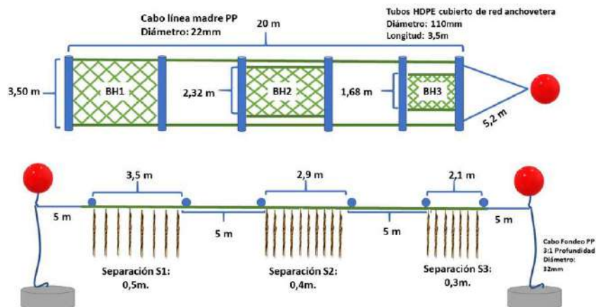
Figura 1: Diagrama de diseño y dimensionamiento del modelo BIVALNET® horizontal para el cultivo de huiro flotador ( Macrocystis pyrifera ) en Punta Trana, Golfo de Arauco. Fuente: Elaboración propia.
