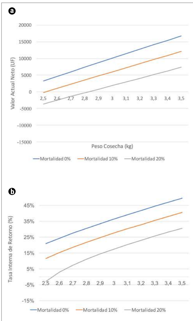
Figura 5: (a) Valor Actual Neto (VAN) en Unidades de Fomento (U.F.) y (b) Tasa Interna de Retorno (%) según peso de cosecha y porcentajes de variación de la mortalidad de Macrocystis pyrifera cultiva con sistema BIVALNET® horizontal.
