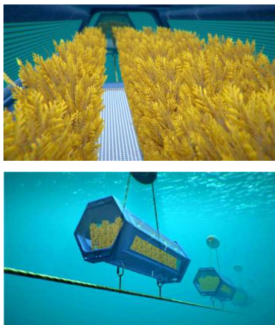
Figura 3: Vistas externas e internas (con sustrato tipo algas inertes para brindar refugio a larvas y alta superficie de adhesión a biopelícula) de un dispositivo Aqvanursery dispuesto en mar.
