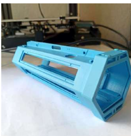
Figura 6: De izquierda a derecha: i) dispositivos renderizados en 3D, ii) taller de fabricación de prototipos mediante impresión 3D, iii) dispositivo Aqvanursery® impreso en 3D.
