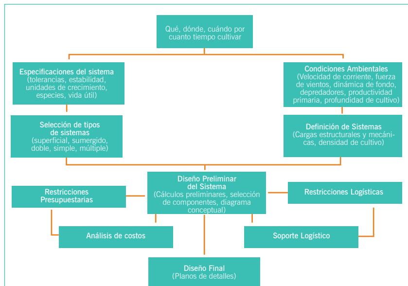
Figura 1. Metodología para el diseño y dimensionamiento de un sistema de cultivo de pequeña escala (modificado de Berteaux, 1976).
