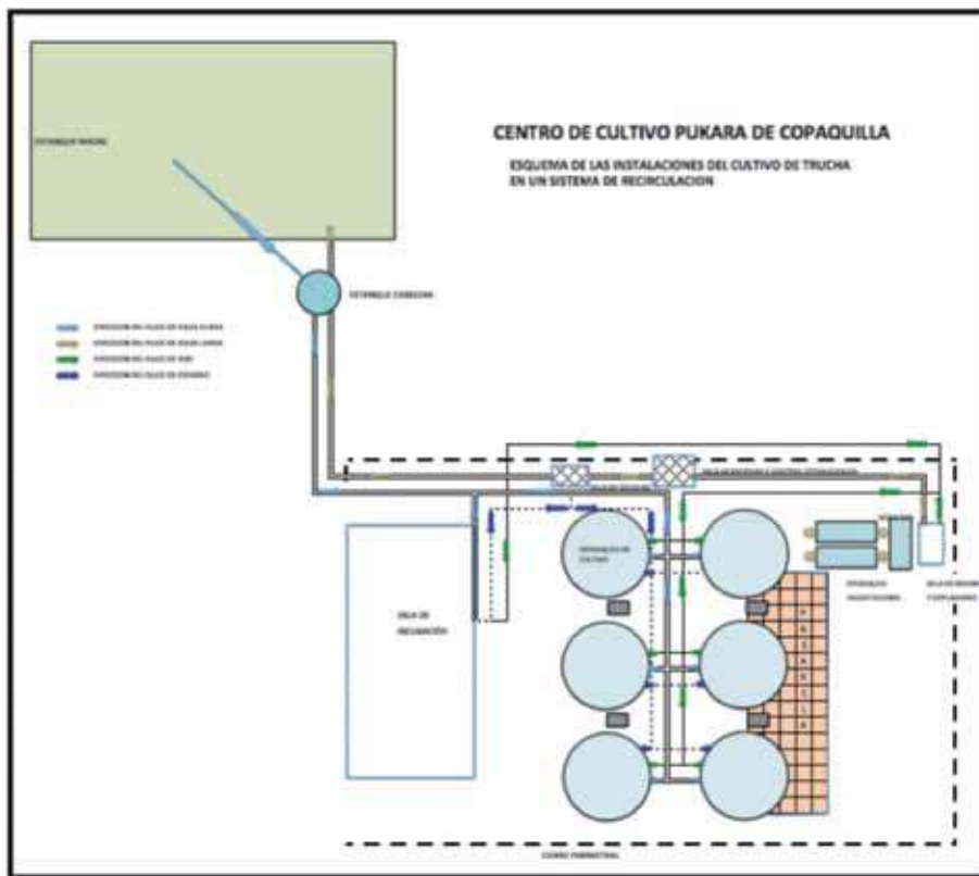
Figura 4. Layout de las instalaciones del cultivo de truchas en recirculación.
