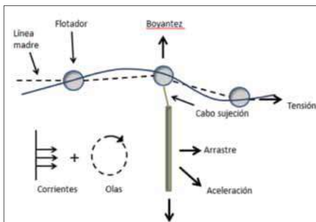
Figura 2. Diagrama de cuerpo libre de elementos estructurales representando los flotadores conectados y las unidades de crecimiento mediante un cabo de sujeción. (Fuente: Modificado de Stevens et al., 2008).
