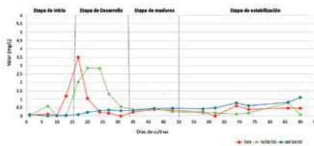
Figura 3. Representación gráfica de las etapas de la formación, desarrollo y estabilización de un sistema de cultivo con tecnología Biofloc. Esquema de elaboración propia a partir de antecedentes registrados durante las actividades del proyecto Fondef ID15110353.
